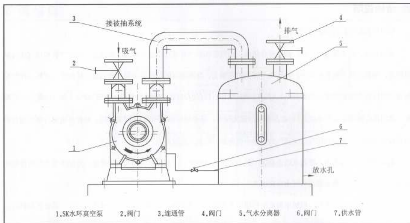
图5 SK水环泵系统示意图
