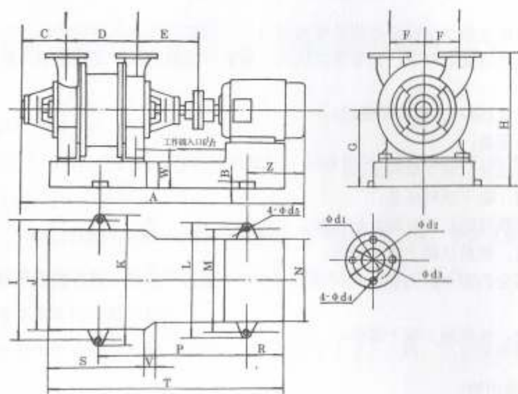
SK-1.5、SK-3外形及安装尺寸
