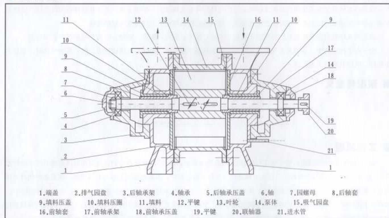
图3 SK-1.5/3水环泵
