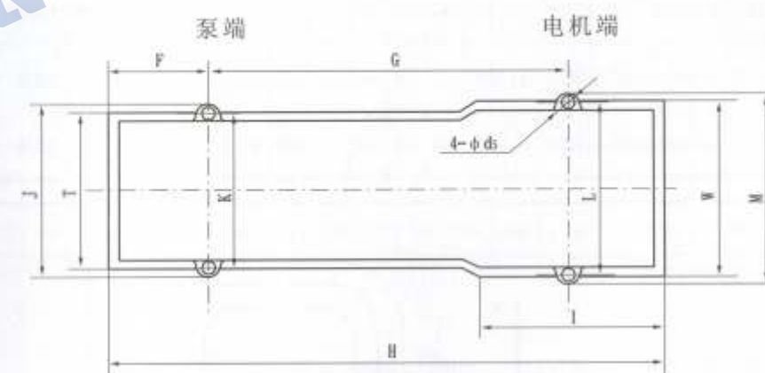
SK-6、SK-12、SK-20、SK-20B底脚安装尺寸 及SK-30、SK-30B真空泵底脚安装尺寸
