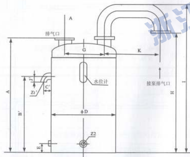
SK-6、SK-12、SK-30水环真空泵气水分离器外形尺寸 SK-20、SK-42气水分离器与SK-30外形尺寸通用 SK-20B、SK-30B、SK-42B气水分离器与SK-30外形尺寸通用
