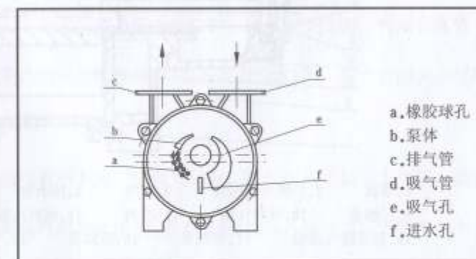
图2 水环真空泵及压缩机结构图
