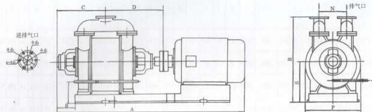
SK-6、SK-12、SK-20、SK-20B、SK-30、SK-30B、SK-42、SK-42B 真空泵及压缩机外形及安装尺寸
