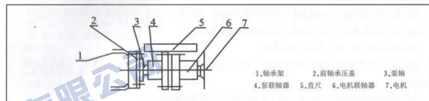
图6 同心度校正方法
