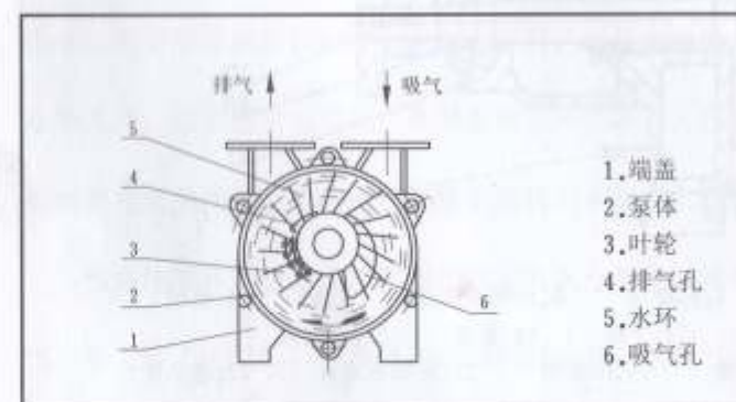
图1 水环真空泵及压缩机工作原理图
