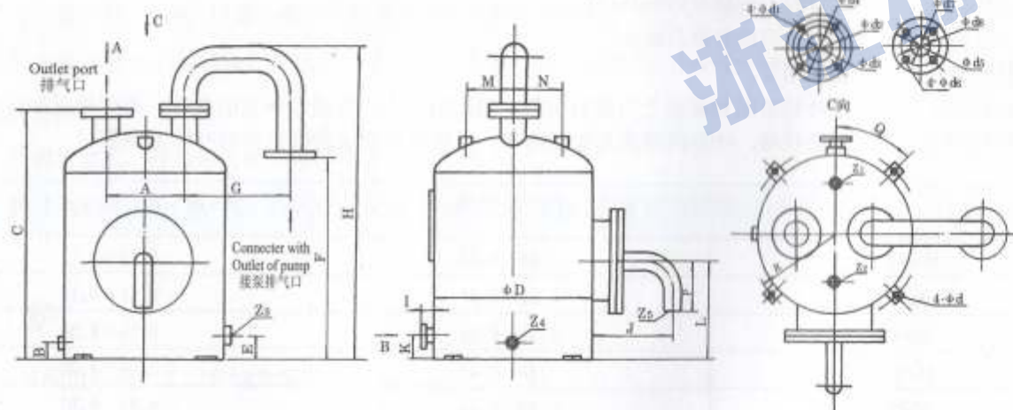
SK-1.5、SK-3水环真空泵及压缩机用气水分离器外形及安装尺寸
