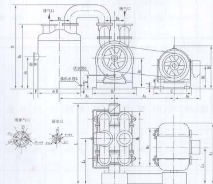
SK-60、SK-85、SK-120水环泵外形及安装尺寸
