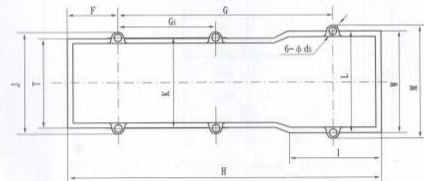
SK-30压缩机及SK-42、SK-42B真空泵底脚安装尺寸
