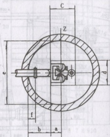
双导轨单泵排水平面图
